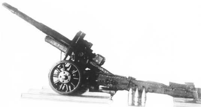
152-мм гаубица-пушка МЛ-20 образца 1937 г.
