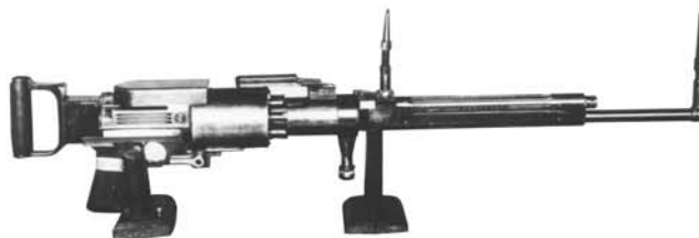
7,62-мм авиационный скорострельный пулемет системы Шпитального-Комарицкого ШКАС образца 1930 г.
