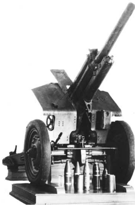
122-мм гаубица М-30 образца 1938 г.
