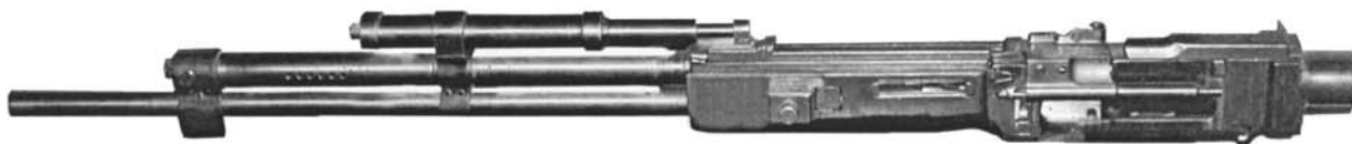
12,7-мм авиационный универсальный синхронный пулемет системы Березина УБС образца 1941 г.
