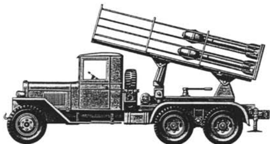
Реактивная система БМ-31-12
