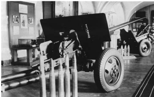
57-мм противотанковая пушка ЗИС-2 образца 1943 г.
