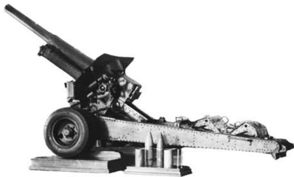
152-мм гаубица образца 1938 г.
