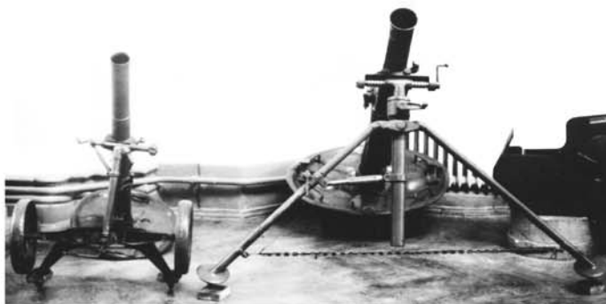
82-мм и 120-мм миномёты образца 1943 г.
