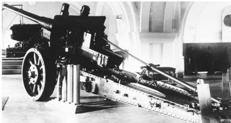
122-мм пушка А-19 образца 1931/1937 г.
