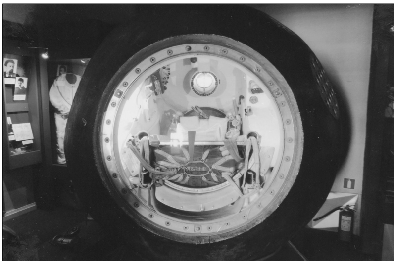
Спускаемый аппарат космического корабля «Восток»
