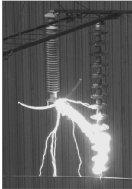
Испытание ОПН-ЛИр-220
