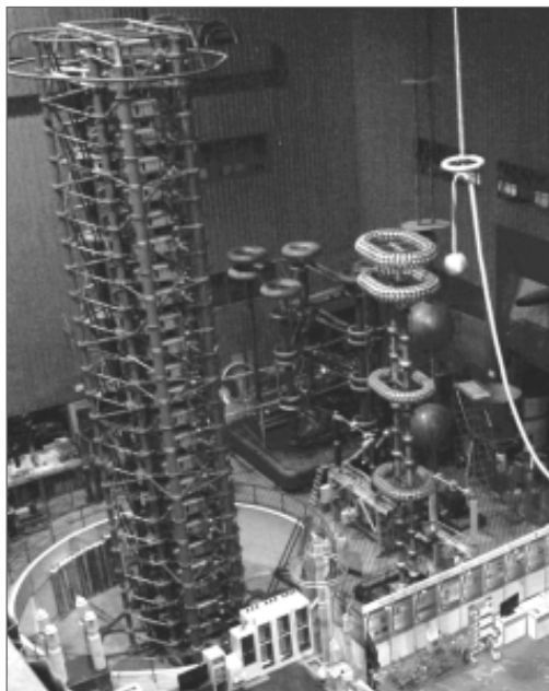
Генератор импульсных напряжений ГИН-6,0 МВ
