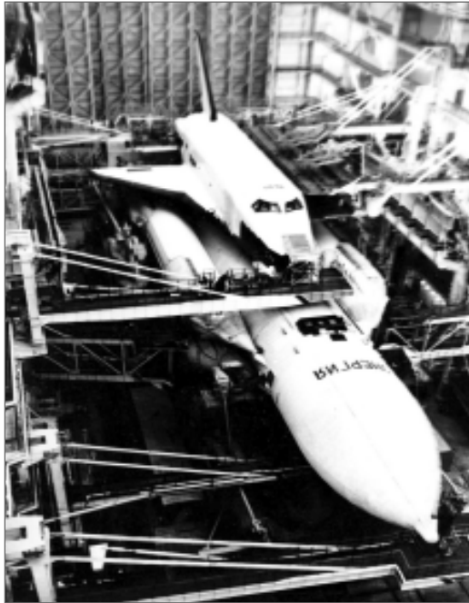
Космический комплекс «Энергия» в сборочном цехе на Байконуре
