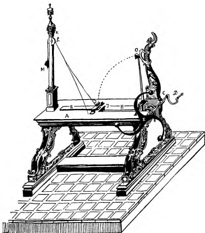
Зубонасекальный станок для производства напильников: по рукописной книге Нартова «Ясное зрелище машин».
