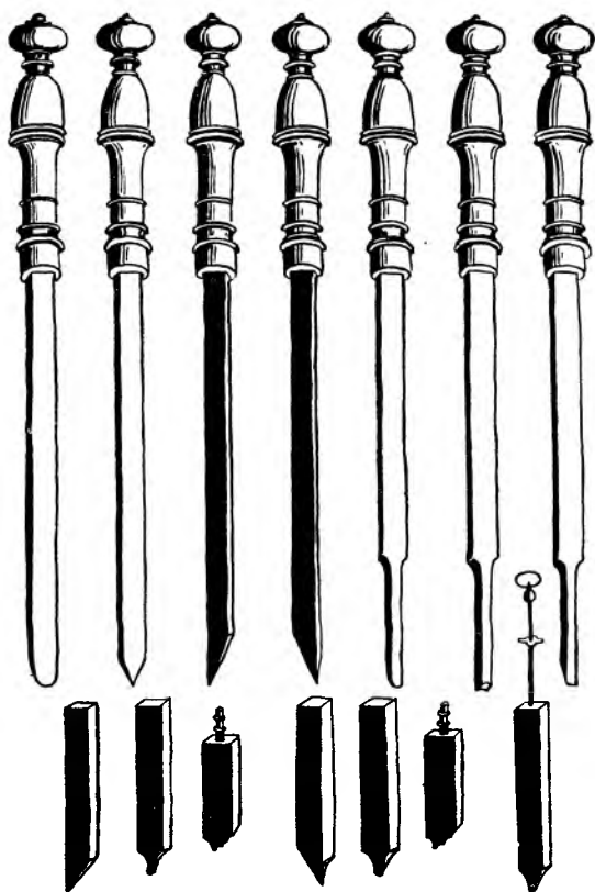
Токарные резцы. По рукописной книге А. К. Нартова «Ясное зрелище машин».
