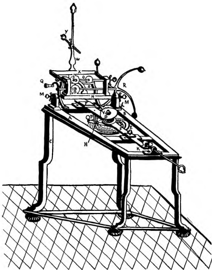
Фрезерный станок для нарезания зубчатых колес: по рукописной книге Нартова «Ясное зрелище машин».
