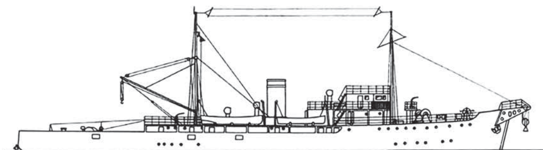
Спасательное судно «Нептун». Спущено на воду 23 февраля 1939 г., вошло в состав плавсредств ЭПРОН 28 декабря 1940 г. С началом Великой Отечественной войны включено в состав аварийно-спасательных сил Краснознаменного Балтийского флота
