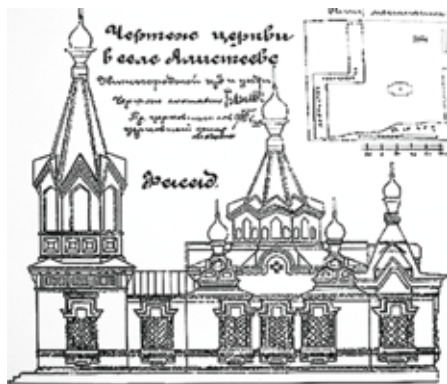
■ Чертёж церкви в Алистево
