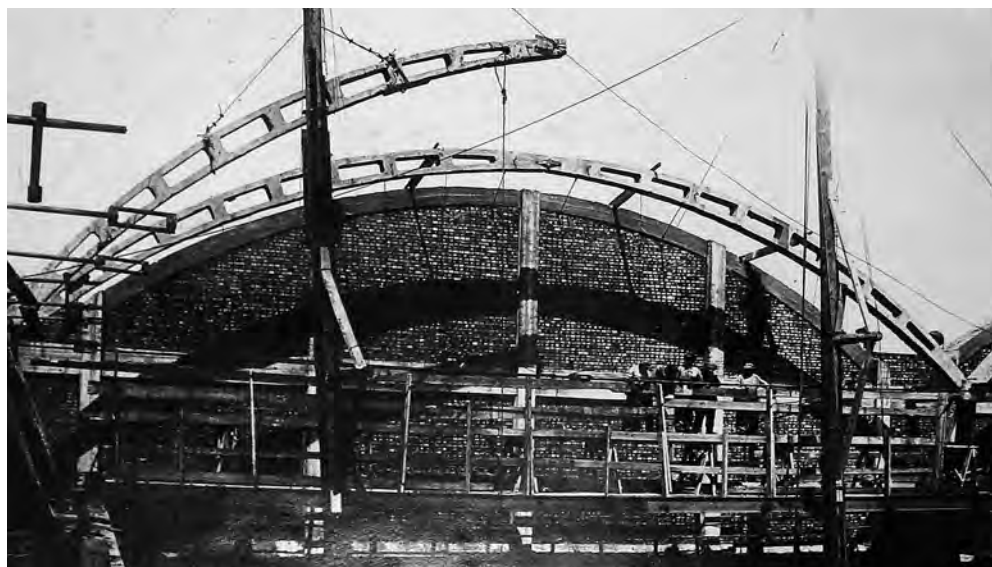
Монтаж крыши завода. 2 августа 1935 // Из фондов музея истории завода «Химпром». Крыша делалась из стекла, чтобы в случае аварии взрывная волна направлялась вверх, сохраняя стены и внутренние помещения
