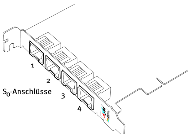
Die Nummerierung der S_0 -Anschlüsse des Controllers C4
