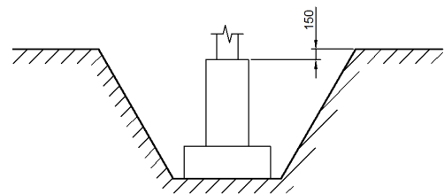
Рис. 77. Фундамент «нулевого цикла» (сначала засыпают котлован, затем монтируют колонны)
