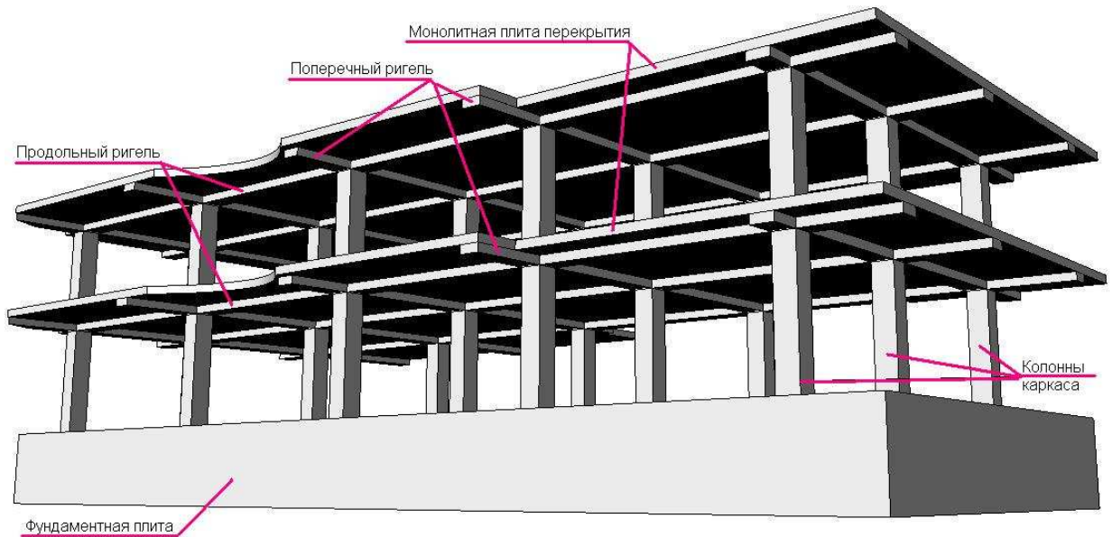
Схема устройства монолитного ригельного несущего остова
