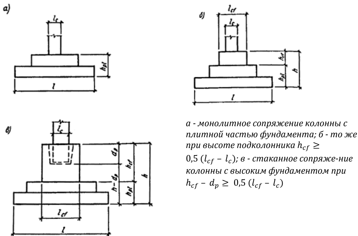
Рис. 79. Виды сопряжений фундамента с колонной по 1-й схеме расчета на продавливание [64]
