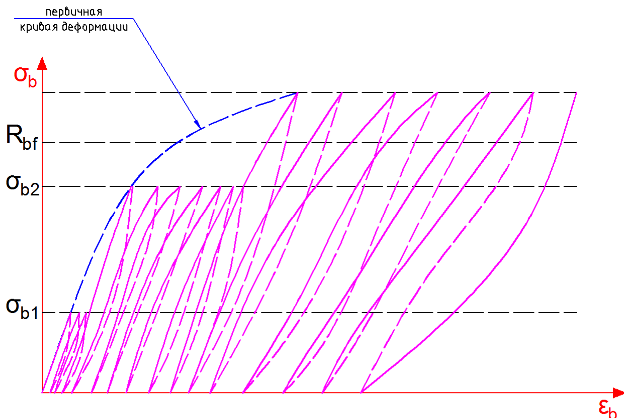
Рис. 20. Диаграмма \sigma - \varepsilon при многократно повторяющихся нагрузках
