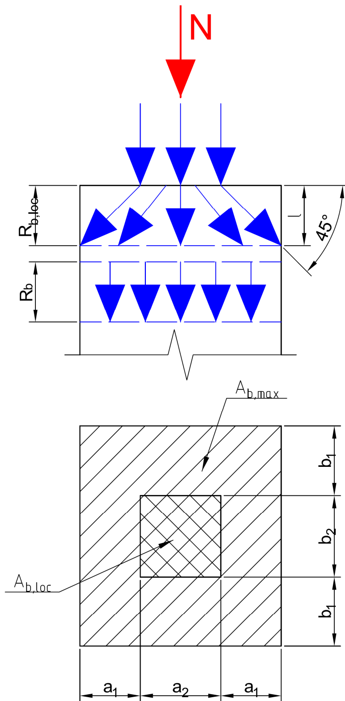
Рис. 14. К определению прочности бетона на смятие
