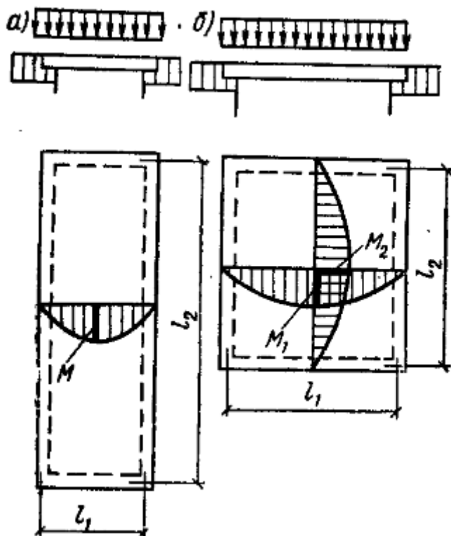
Рис. 68. Работа плит перекрытия в зависимости от соотношения сторон [1]
