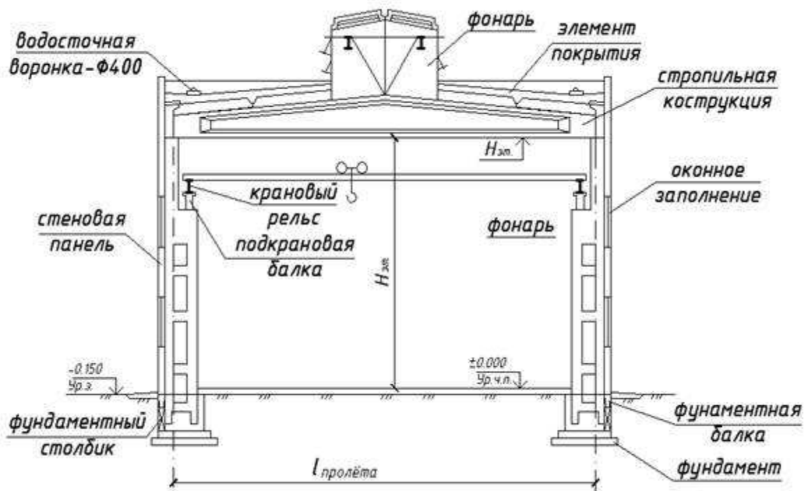
Рис. 44. Разрез одноэтажного промышленного здания [31]
