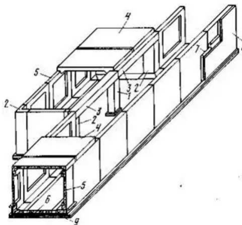
Рис. 91. Камера сборного железобетонного коллектора: 1 — колонна; 2 — угловой блок; 3 — балка перекрытия; 4 — плита перекрытия; 5 — стеновой блок; 6 — блок днища; 7 — гидроизоляция; 8 — защитная стенка; 9 — двухслойная подготовка из щебня и бетона [65]
