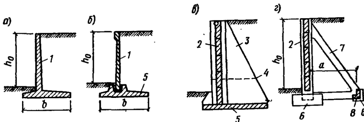
Рис. 92. Конструктивные схемы сборных подпорных стен а- угловая одноэлементная; б- угловая двухэлементная; в- с контрфорсами; г- анкерная; 1 - сборные цельные блоки; 2- стеновые плиты; 3- сборный контрфорс; 4- стык сборных элементов контрфорса; 5- фундаментная плита; 6- опоры рамы; 7- рамы; 8- анкерная балка [1]
