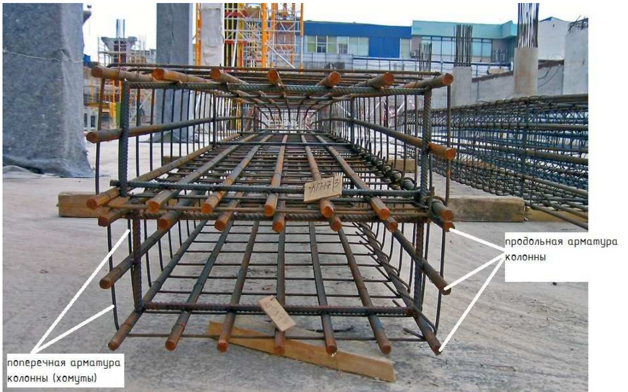
Рис. 25. Армирование колонны [21]
