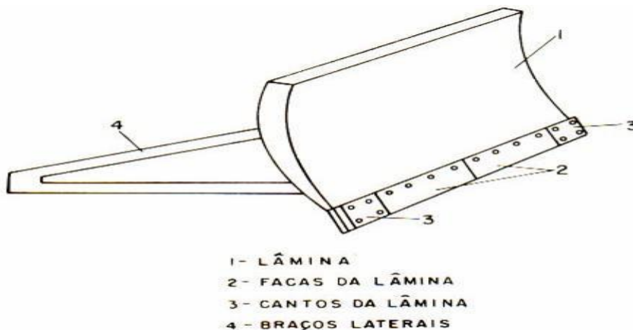
Figura 1 – Lâmina e seus componentes
