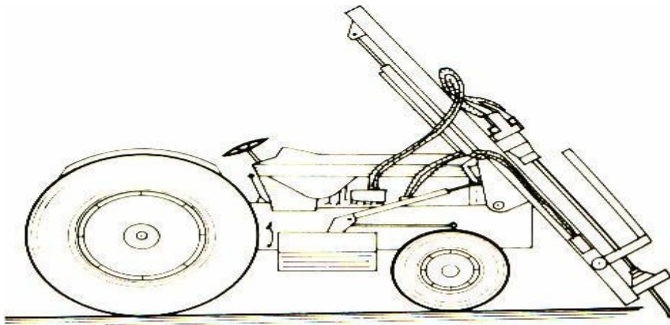
Figura.10 – Perfuratriz com avanço montada sobre trator de pneus
