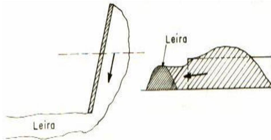
Figura 2 – Trabalho com lâmina não perpendicular ao eixo da máquina
