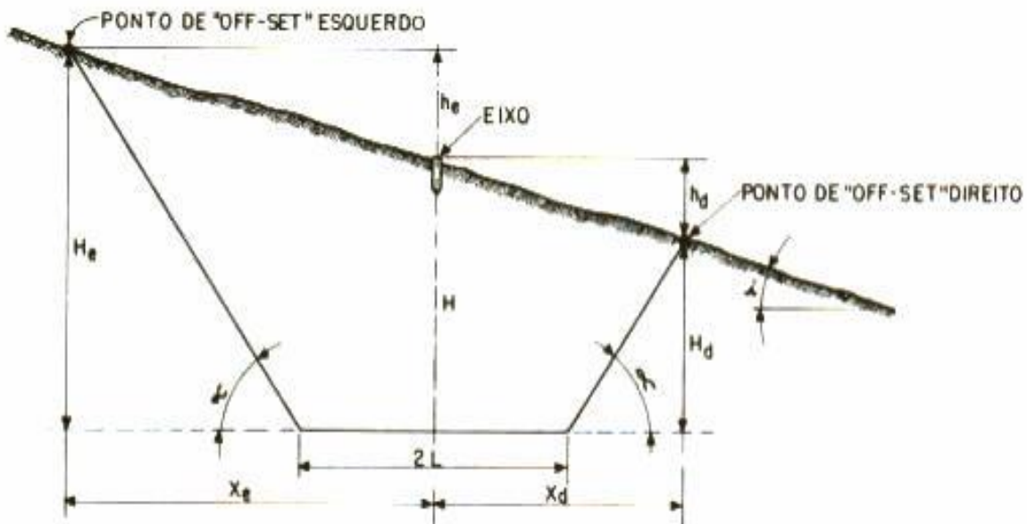
Figura.9 – Elementos para localização dos cortes
