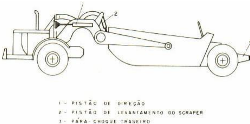
Figura.3 – “Motoscraper” com rebocador de um eixo
