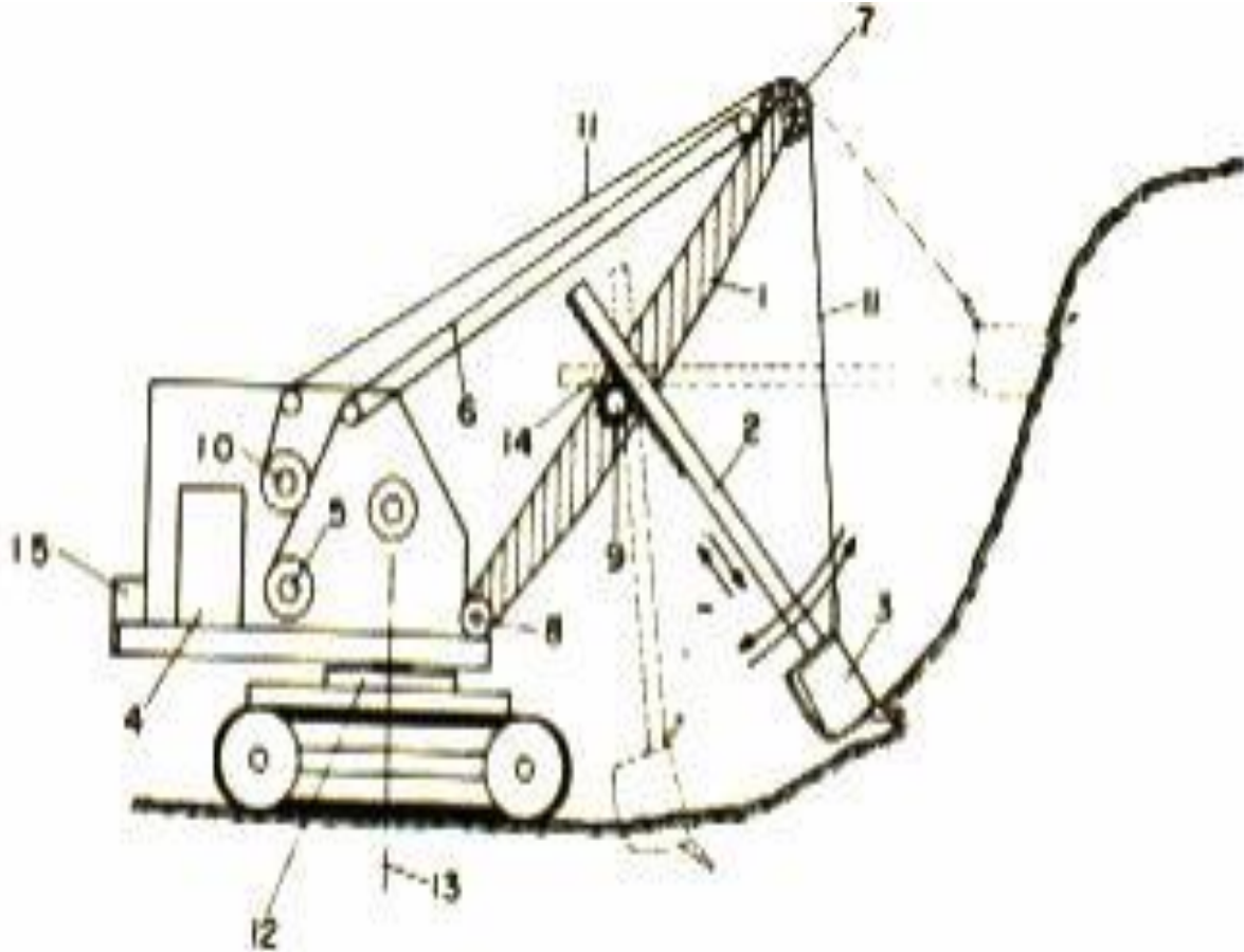
Figura.5 – Escavadeira com lança “shovel
