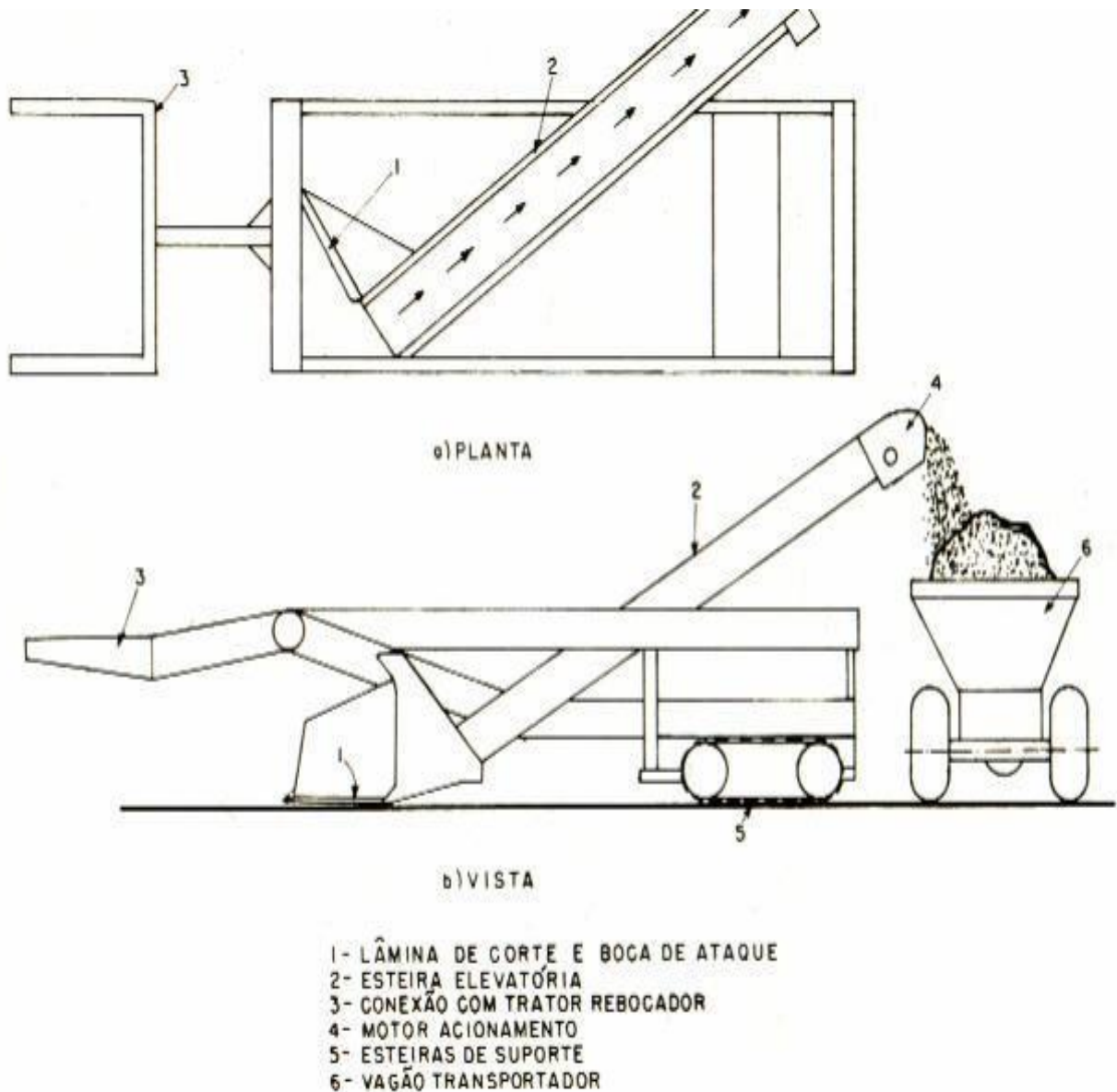
Figura.8 – Unidade escavo-elevadora
