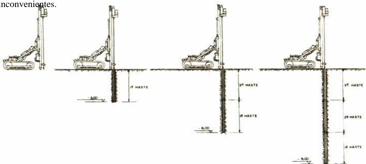
Figura.11 – Sequência de utilização das hastas na perfuração com brocas de extensão
