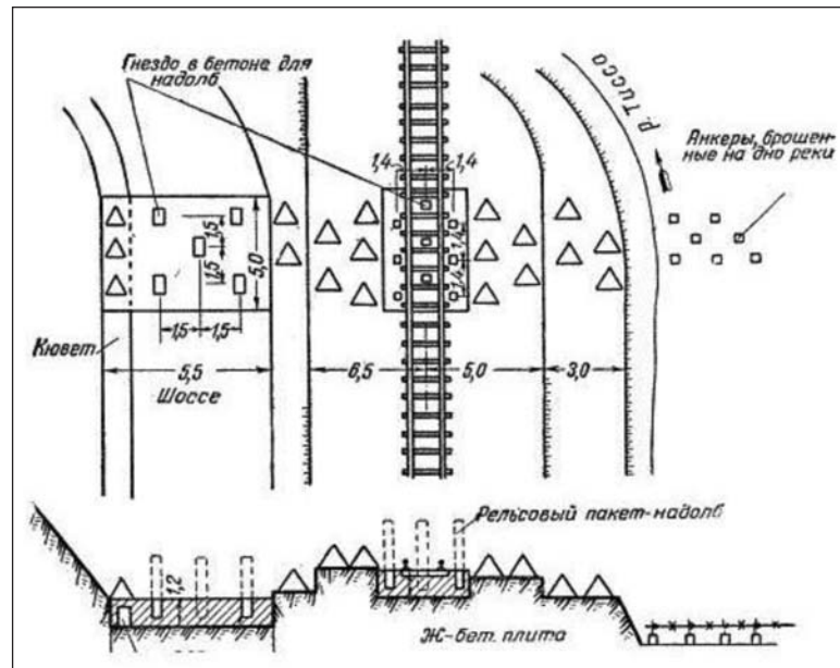
Мал. 9. Пакеты-надолбы [4, рис. 9.]
