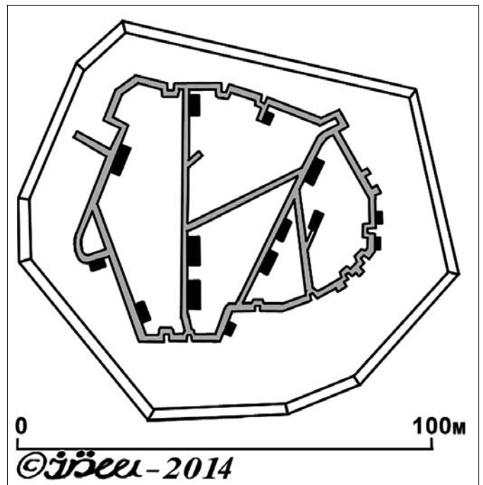
Мал 4. Укріплення типу «Infanterie stutzpunkt», періоду 1908-13 рр. На підставі обмірів опорного пункту Миколаїв-Розвадівського тет-де-пону.
