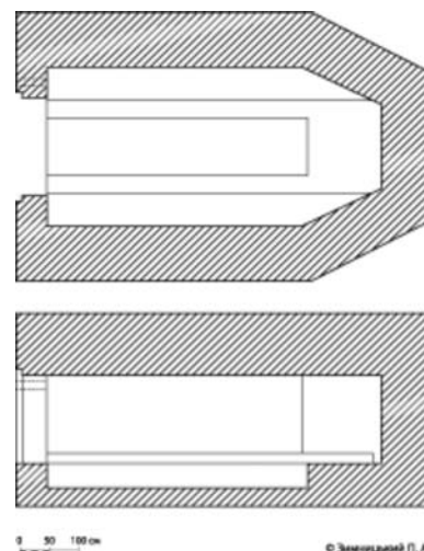
Мал. 7. Схема сховища для протитанкової гармати
