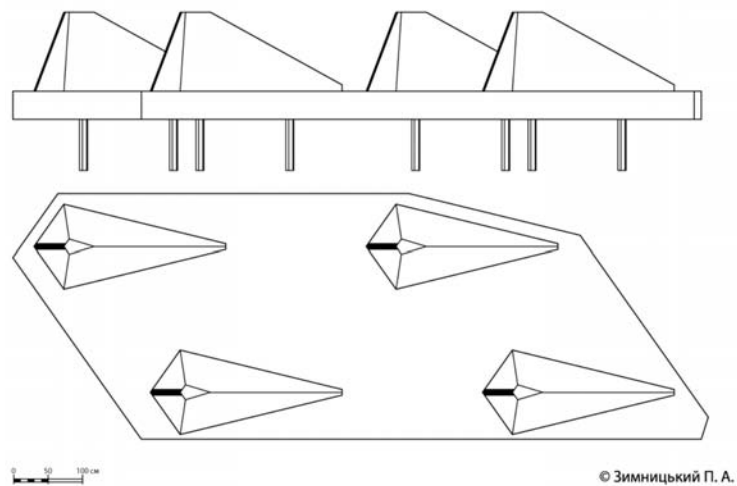
Мал. 2. Протитанкові надовби гідродинамічної форми.
