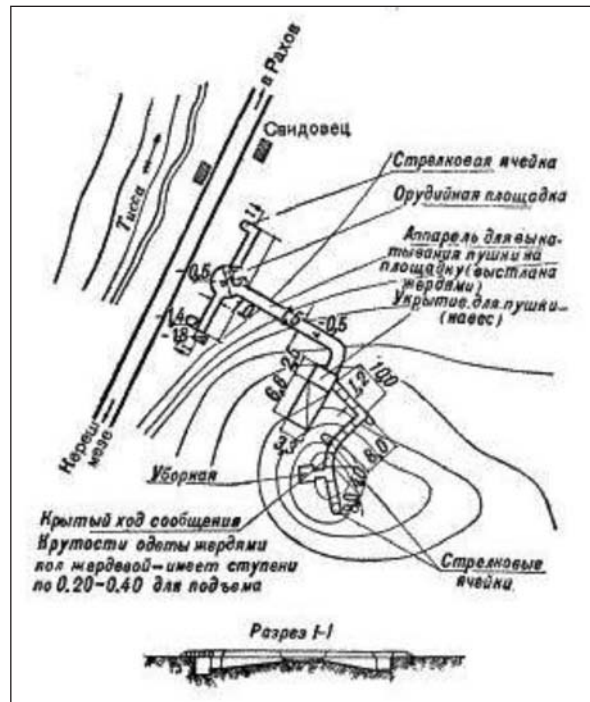
Мал. 8. Артиллерийская позиция [4, рис. 4.]
