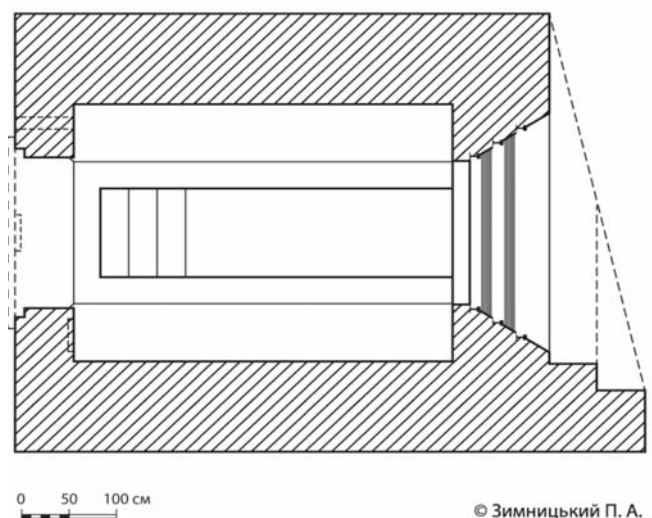
Мал. 4. Схема артилерійської довготривалої вогневої споруди для стрільби з протитанкової гармати.
