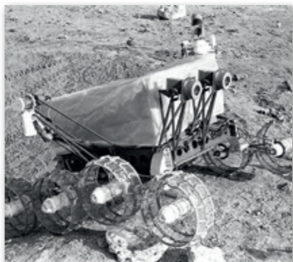
Испытания ходовой части планетохода «Луноход-1» в наземных условиях, имитирующих лунный грунт, на лунодроме Центра дальней космической связи. Крым. Январь 1971 года. Фото Николая Акимова. ТАСС
