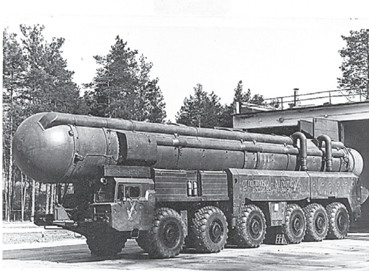
Самоходная пусковая установка 15У106 ПГРК «Пионер»
