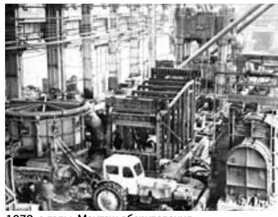
1970-е годы. Монтаж оборудования в кузнечном производстве
