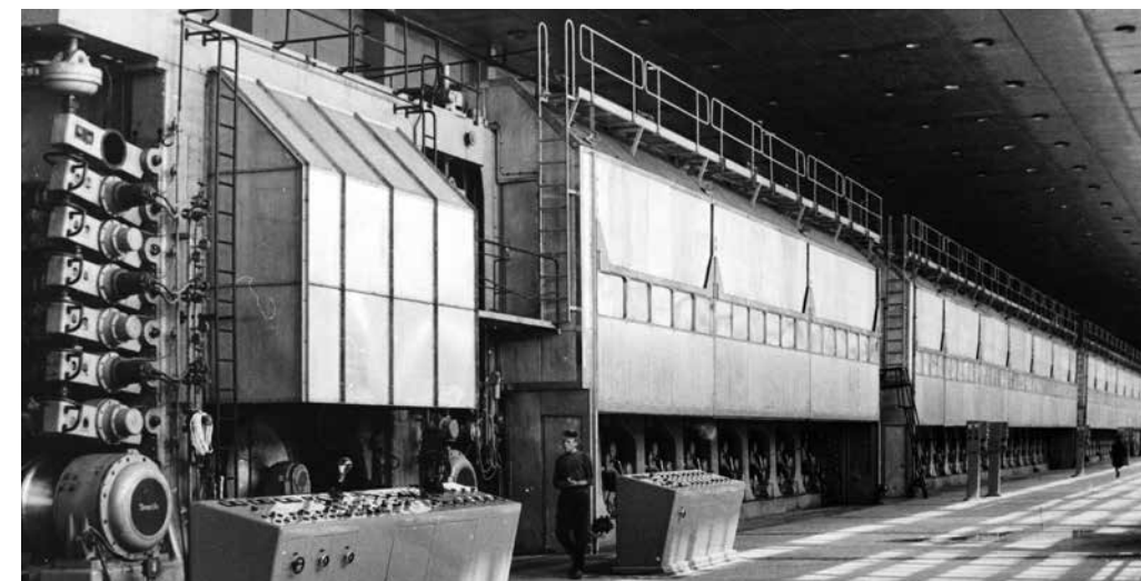
Картоноделательная машина производительностью 820 тонн тарного картона в сутки. Обрезная ширина – 6300 мм
