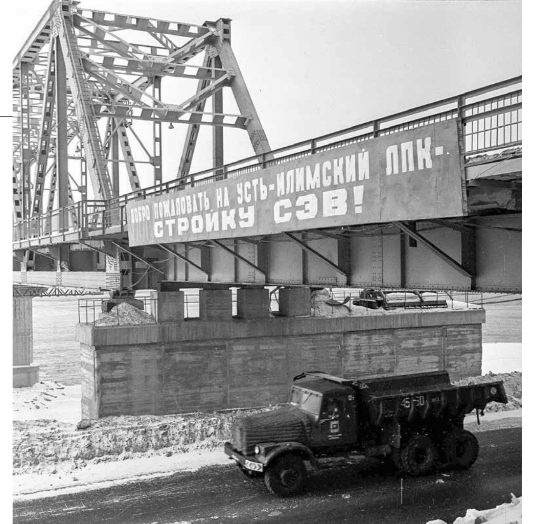
Быстрыми темпами заканчивается строительство моста через Ангару, без которого невозможно разворачивать работы на ЛПК. Его строительство ведет дорожный участок, возглавляемый П.П. Ющенко. Работой руководит опытный инженер-«мостовик» О.А. Белов
