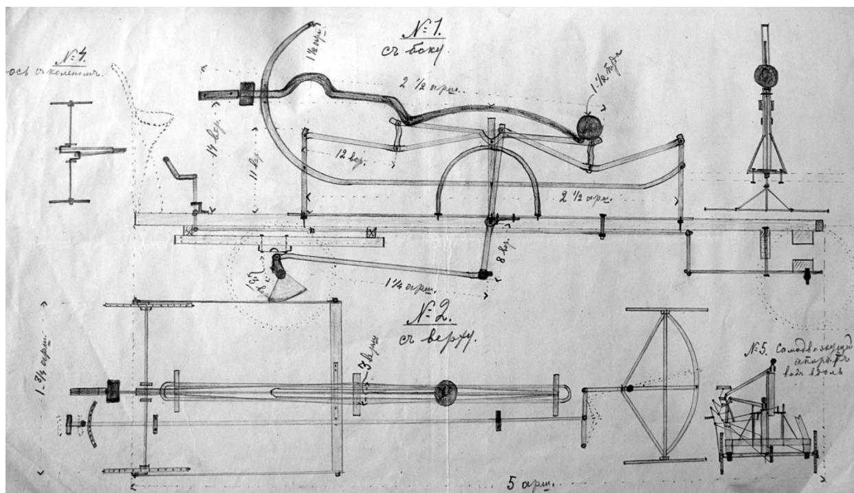
Рис. 1. Схематический рисунок «самодвижущегося экипажа» П.Г. Лысенкова. 1901 г.
