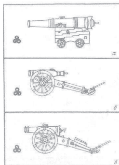
Орудия Динабургской крепости в период войны 1812 года. а - крепостная 24-фунтовая пушка образца 1805 года, вес около пяти тысяч килограммов
