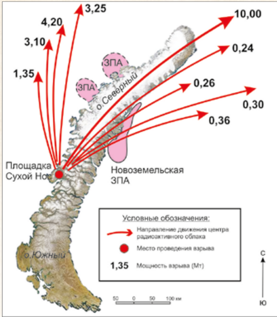
▲ Карта ядерных взрывов
