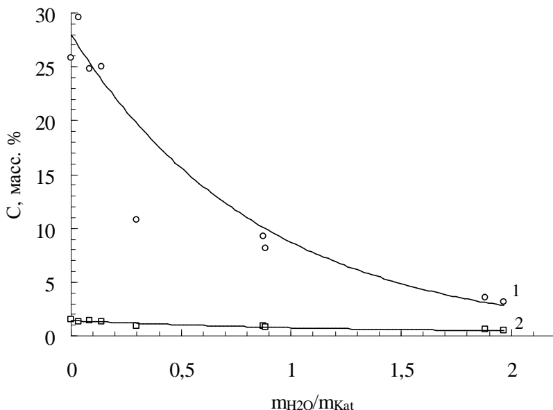
Рисунок 2. Концентрации продуктов реакции дегидратации трет-бутанола с н-пропанолом на катионите КУ-2×8 на 4-м часу реакции при различных отношениях массы воды к массе катализатора в начале опыта (1 – пропил-трет-бутиловый эфир, 2 – изобутилен).
