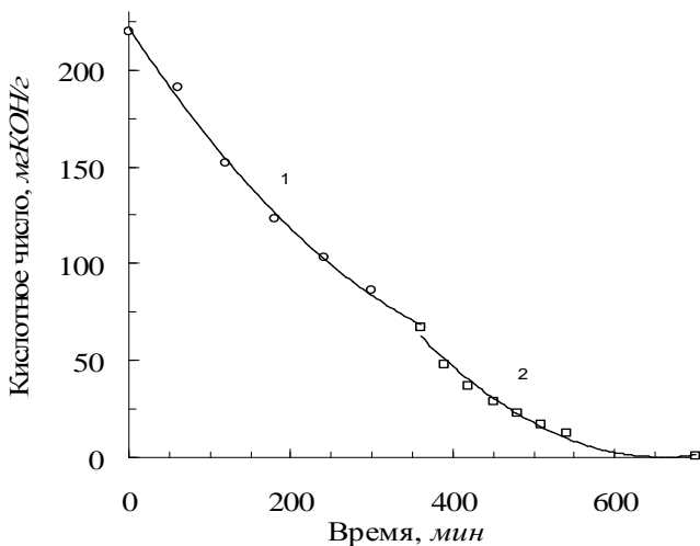
Б 1 - без катализатора. 2 - в присутствии ТМТ
