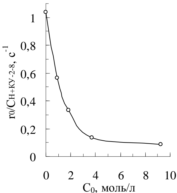
Рисунок 1. Влияние воды на начальную скорость образования пропил-трет-бутилового эфира в реакции межмолекулярной дегидратации ТБ с PrOH
