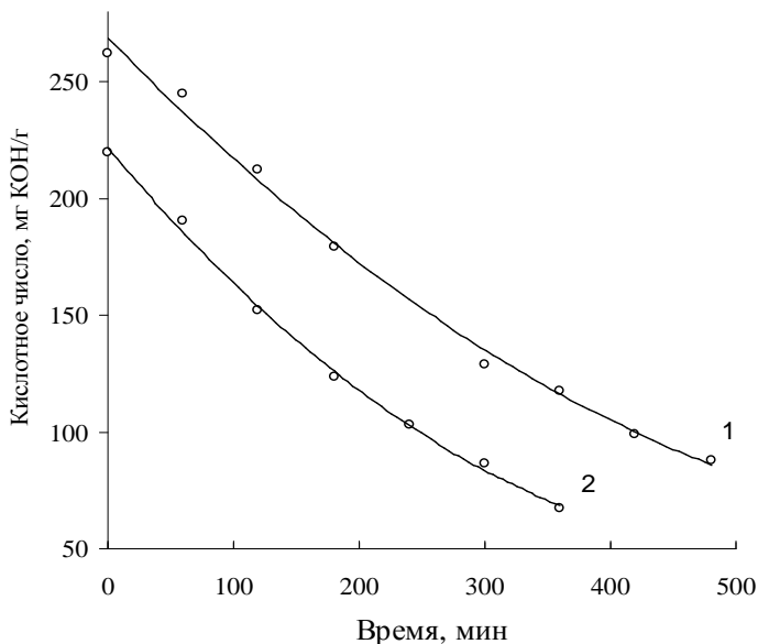
А 1 - диамиладипинат, 2 - дибутиладипинат
