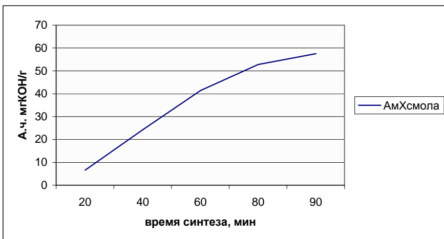
График 1. Зависимость А.Ч. от продолжительности аминирования.
