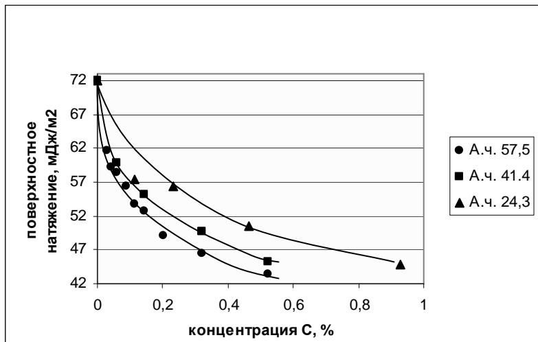
График 2. Зависимость поверхностного натяжения от концентрации.
