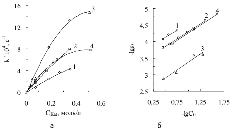
Рисунок 4. Зависимость скорости реакции (1) от концентрации катализатора. а. Зависимость эффективной константы скорости от концентрации КУ-2×8. б. Зависимость начальной скорости реакции от концентрации КУ-2×8. R = 1 – i-Pr, 2 – Pr, 3 – i-Bu, 4 – Bu
