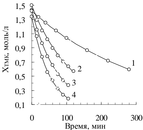
Рисунок 3. Кинетические кривые реакции ВуОН с ТБ на катионите КУ-2-8 при Т (К): 1 – 332, 2 – 342, 3 – 347, 4 – 352 (точки – эксперимент, кривые – расчёт).
