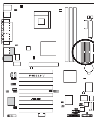
P4B533-V IDE Connectors
