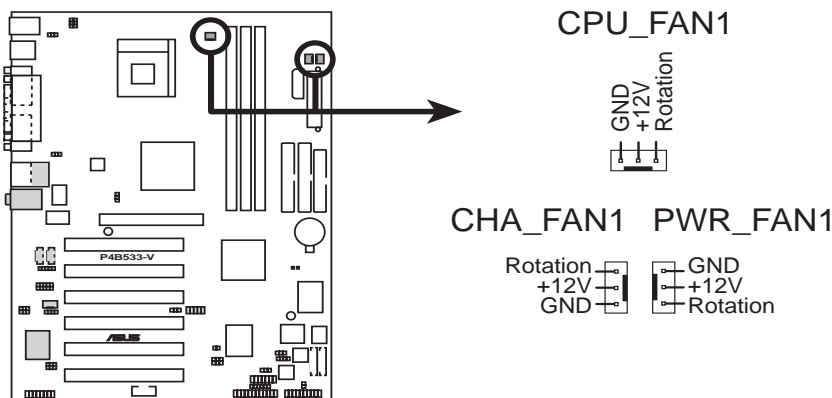
P4B533-V 12-Volt Fan Connectors
