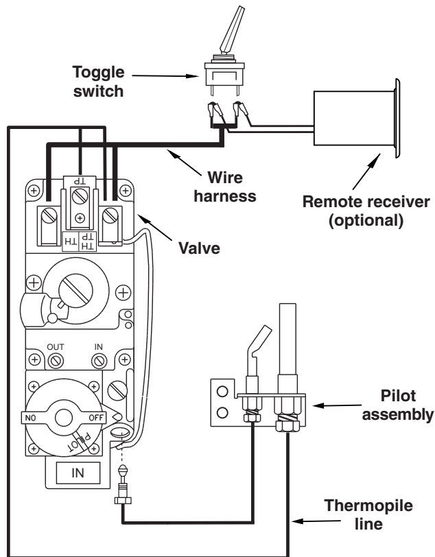
Fig. 10-2
