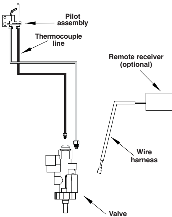
Fig. 10-4
