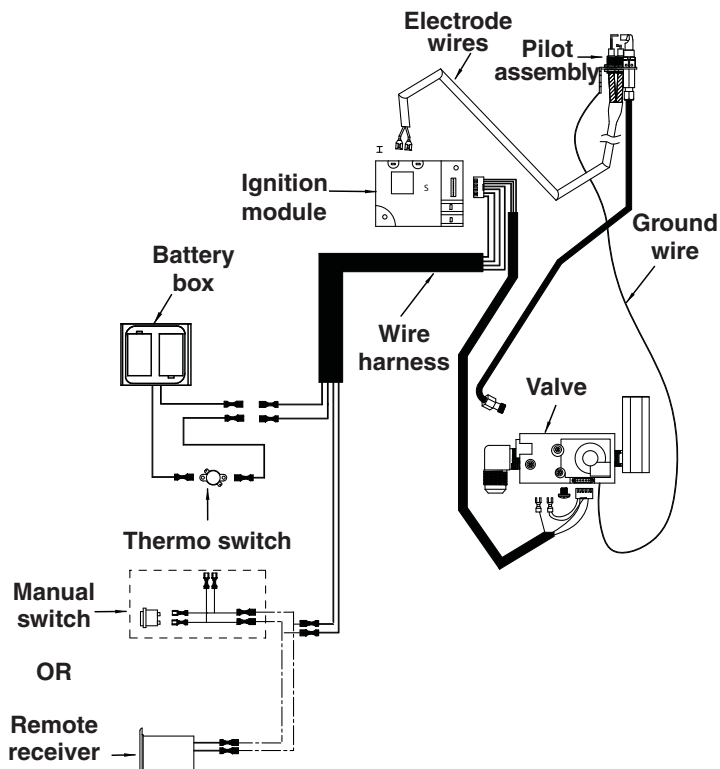
Fig. 10-1
