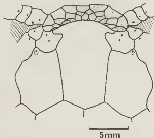
FIG. 7. Pericosmus macronesius Koehler, architecture de la région péristomienne (les interambulacra 1 et 4, hachurés, atteignent le péristome).
